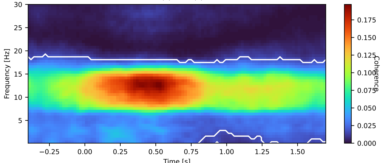
8B (0) - 8AD (2)
